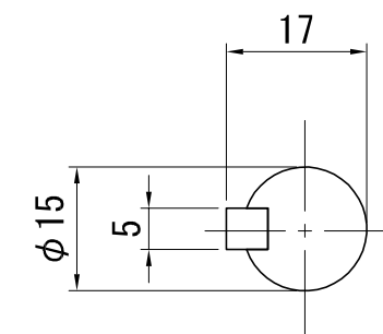
軸端寸法 (1/1)
